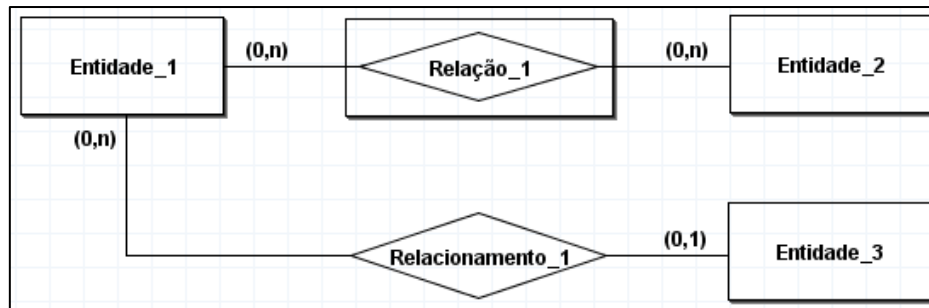
Figura 3 – Esquema conceitual no brModelo 3.3
