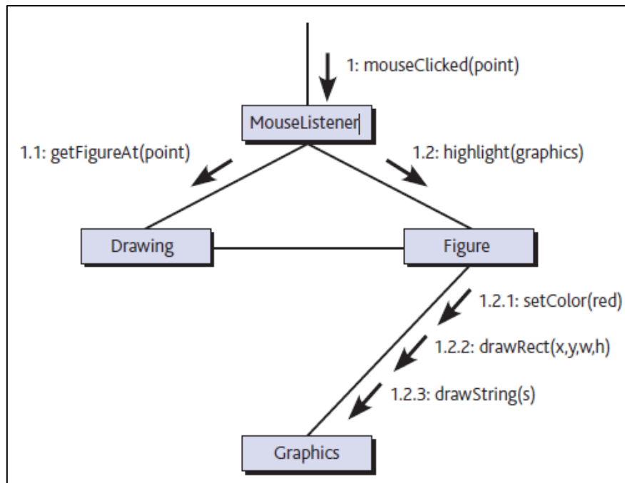
Figura 1 – Diagrama da UML
